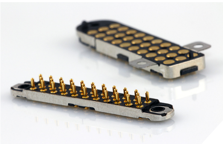
焊接面示意图 (SMT/THT引脚)
